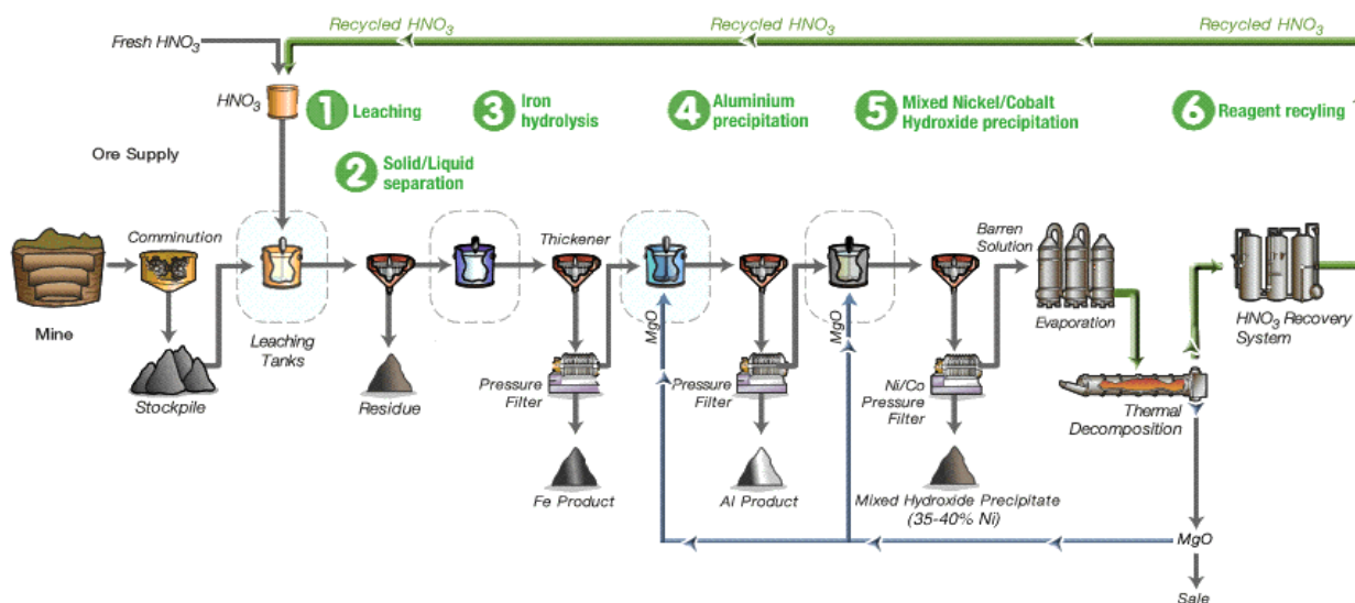
Slika 2 - Direkt Nickel Process [3]
