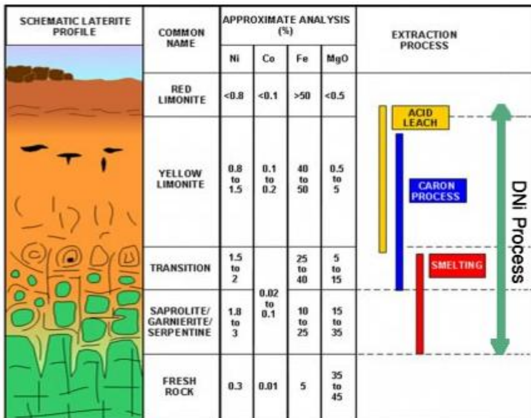
Slika 3 - Primenljivost Direkt Nickel Procesu DNI [3]
