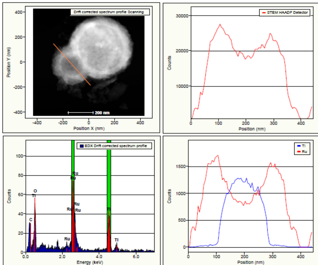
Slika 10 - Idealne "core-shell" čestice rutenijum (IV)-oksida proizvedene na titan-dioksidu
