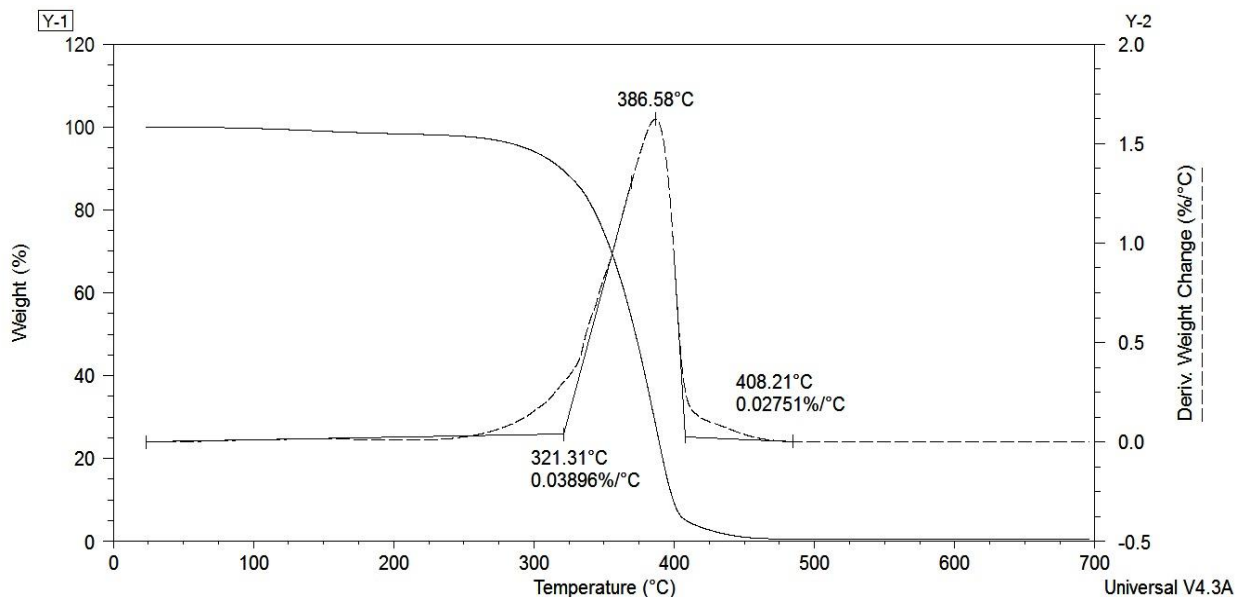
Slika 2. Kriva promene mase uzoraka sa temperaturom (TG) i diferencijalna termogravimetrijska kriva (DTG) pri zagrevanju uzorka brzinom od 5°C/min od sobne temperature do 700°C za uzorak sa 60 mas. % alkidne smole
