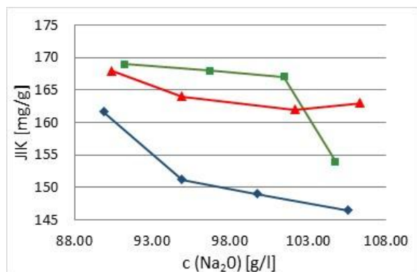
Slika 2. Uticaj koncentracije \text{Na}_2\text{O} na jonoizmenjivački kapacitet za vreme reakcije 60 (◆), 120 (■), i 150 (▲) minuta
